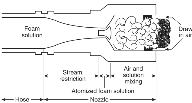
FIGURE 5.3.1.2.1(d) Multifunction Foam Device.
