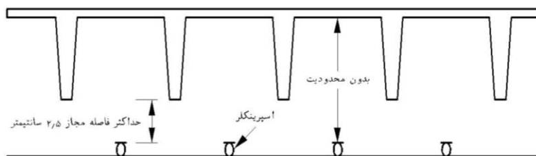
شکل ۱۰-۵-۴-الف-۲- نصب اسپرینکلر در سازه سیمانی T شکل
