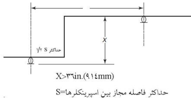
شکل ۹-۵-۴-ب- تغییر عمودی در ارتفاع سقف کمتر یا برابر با ۹۱۴ میلی‌متر (۳۶ اینچ)
