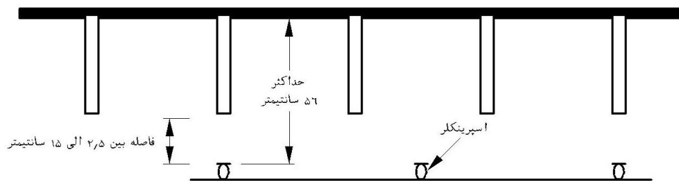
شکل ۱۰-۵-۴-الف-۱- نصب اسپرینکلر در سازه مسدودکننده
